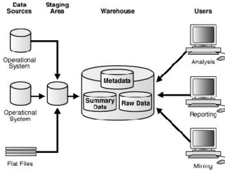
شكل (1) نموذج مستودع البيانات
