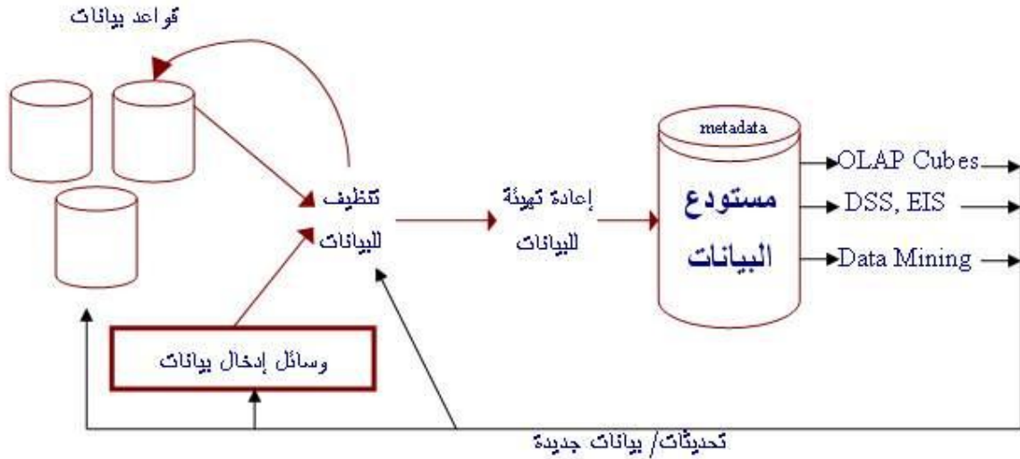
شكل (2) بناء مستودعات البيانات
